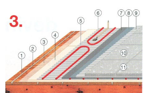
3. Verlegung auf Holzdielen oder Spanplatten
