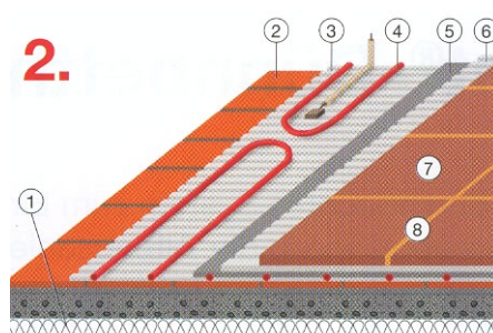
2. Verlegung auf altem Fliesenbelag
