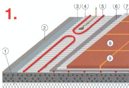
1. Verlegung auf Estrich
